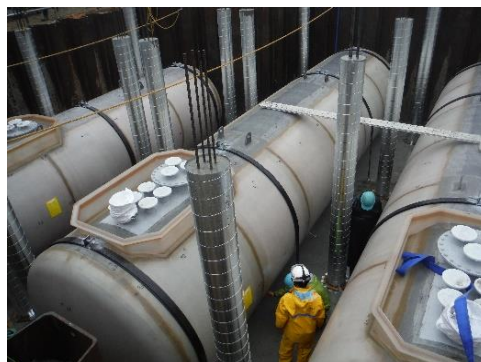
(地下タンク貯蔵所の埋設時現地検査)
